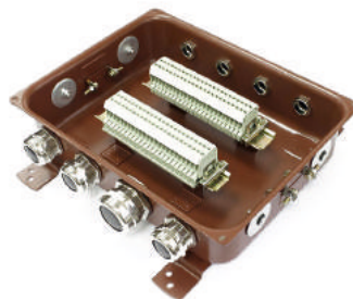
Коробки клеммные
